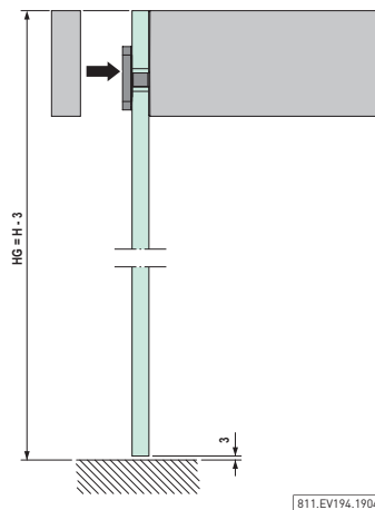
Einbausituationen mit Glaswandhalter
