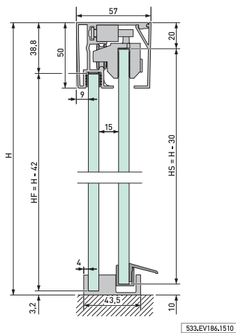
Einbausituationen mit umlaufendem Profil
